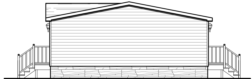
RIGHT ELEVATION
